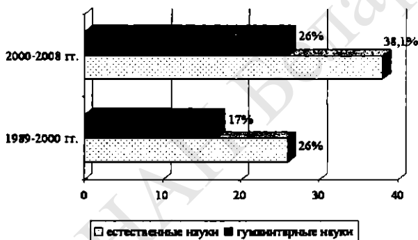
Рис. 1. Активные по степени использования документы в периоды 1989-2000 гг. и 2000-2008 гг.
